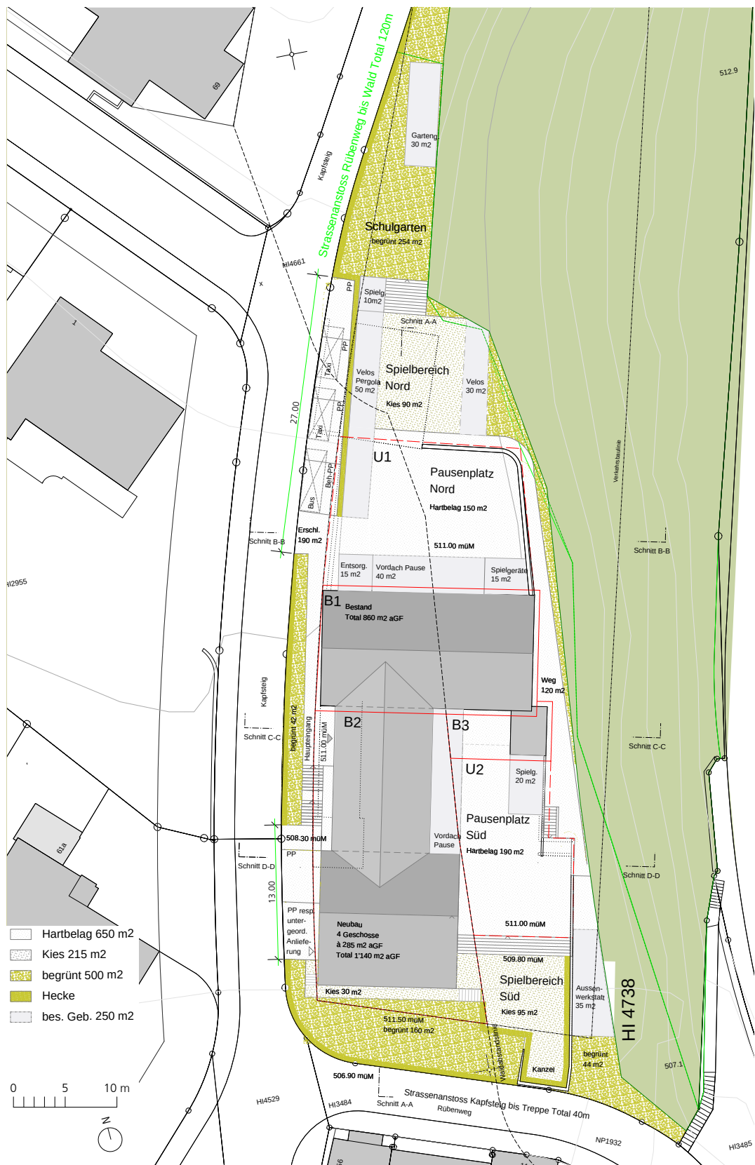
Abb. 20: Situations- und Umgebungsplan Machbarkeitsstudie mit Baubereichen gemäss Gestaltungsplan
