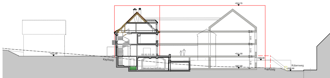
Schnitt A-A
