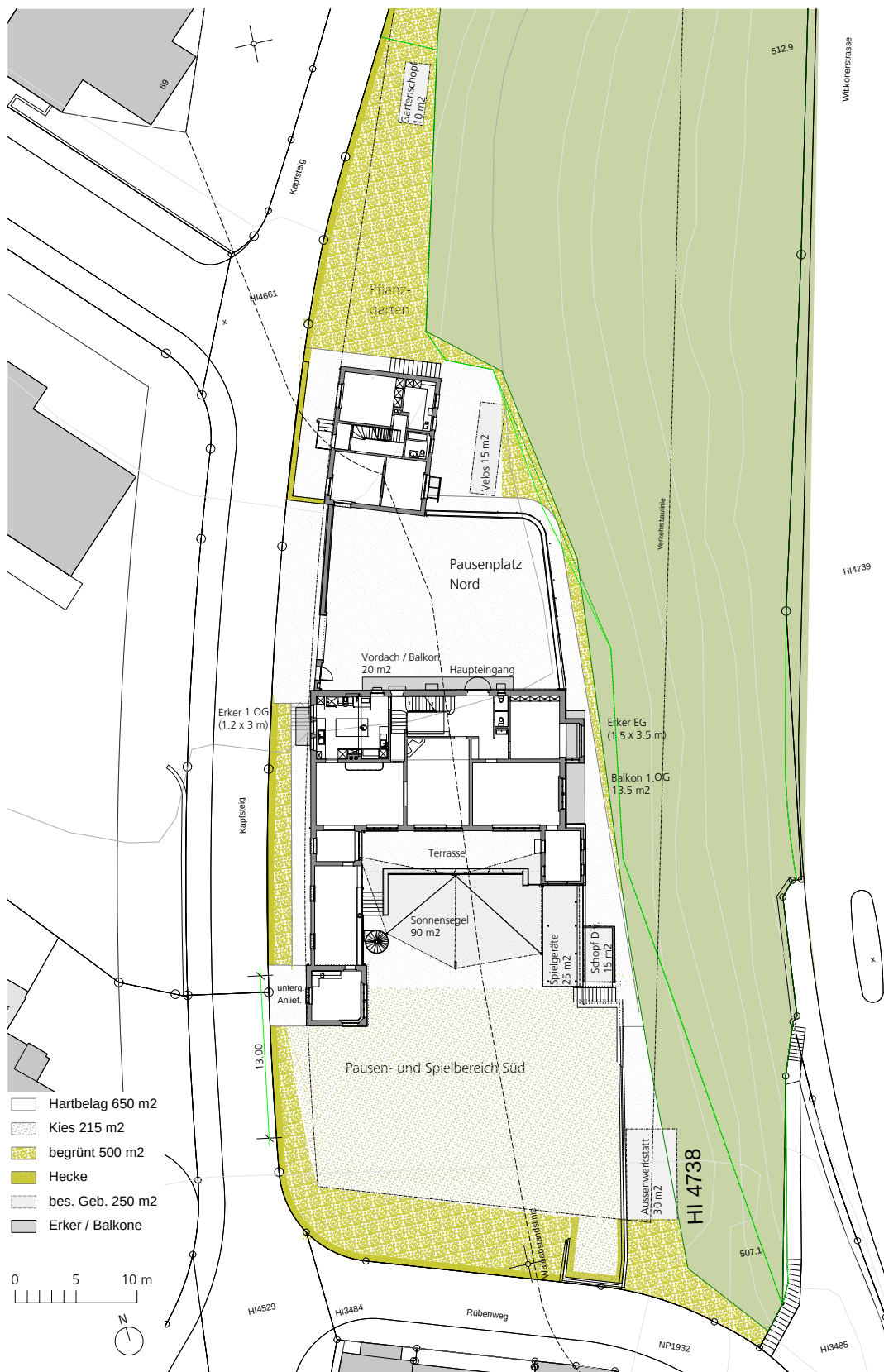
Abb. 16: Ist-Zustand (EG Grundriss) des Bestands sowie die Umgebung mit Pausenbereichen und diversen gedeckten Aussenbereichen
