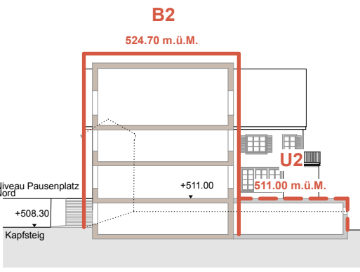
Schnitt D-D
