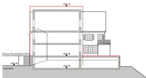
Schnitt D-D
