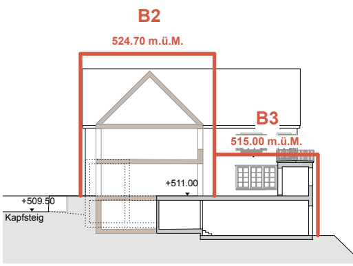
Schnitt C-C
