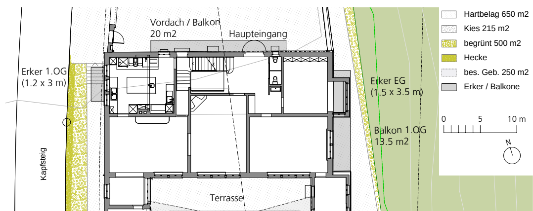
Abb. 15: Planausschnitt Ist-Zustand (EG Grundriss) des Bestands mit Erker und Balkonen
