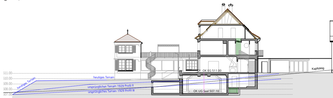
Abb. 12: Der Längsschnitt vom Ist-Zustand zeigt, dass das ursprüngliche Terrain ungefähr der Steigung des Kapfsteigs folgte und die Terrasse im südlichen Bereich des Hauptgebäudes aufgeschüttet wurde.
