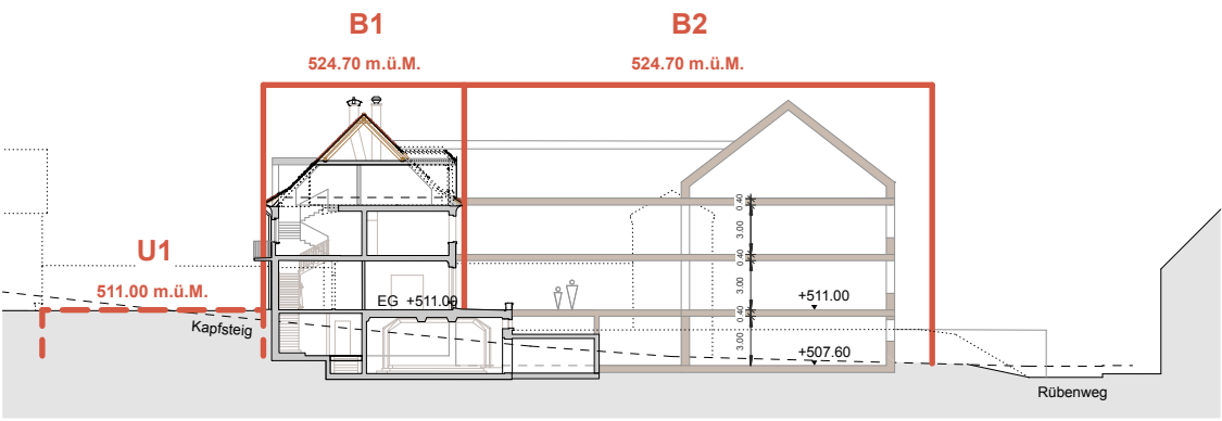
Schnitt A-A
