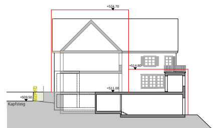
Schnitt C-C
