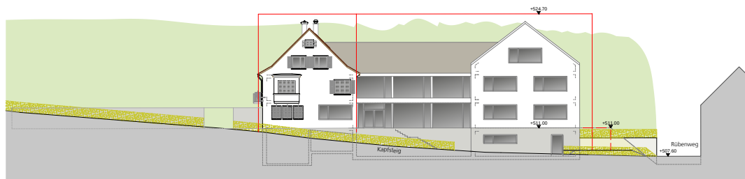
Ansicht West
