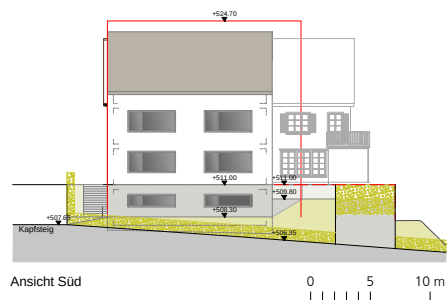
Abb. 21: Schnitte und Ansichten Machbarkeitsstudie mit Baubereichen gemäss Gestaltungsplan
