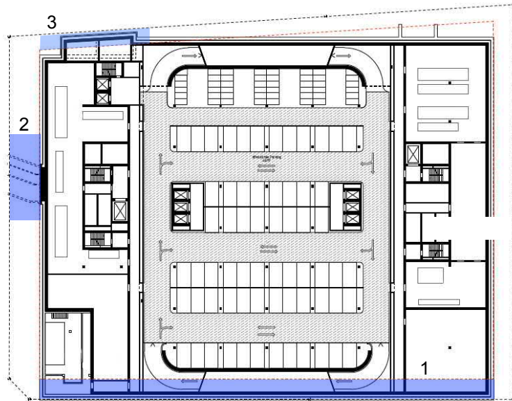
Abb. 9: 2. Untergeschoss gemäss Richtprojekt Stand 04.07.2017
