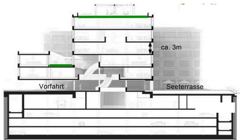
Abb. 8: Schnitt Richtprojekt, Geschosshöhe, Terrassen (grün), Stand 04.07.2017
