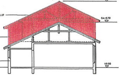
SCHNITT A-A 1:100
