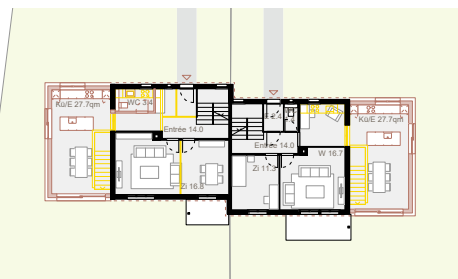
Untergeschoss
