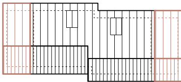
Dachaufsicht
