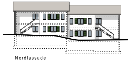
Nordfassade
