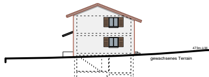
Ostfassade
