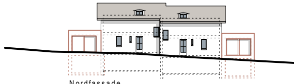
Nordfassade
