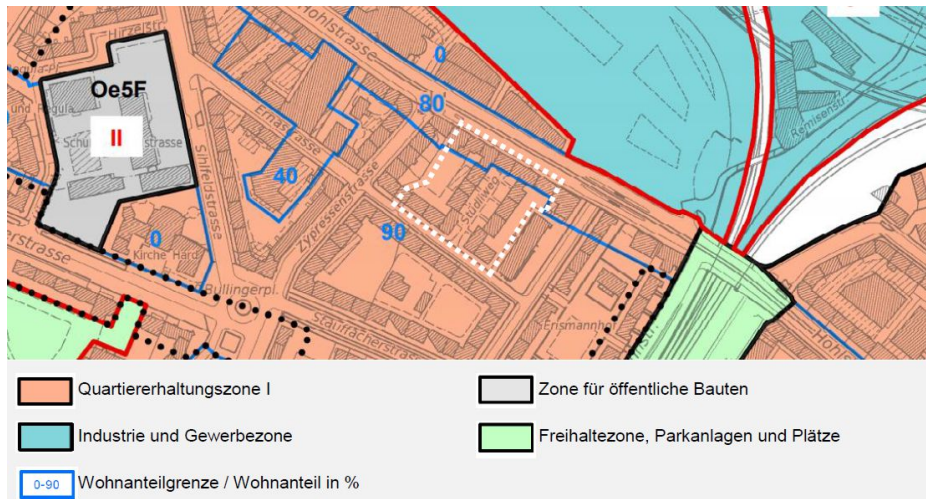
Abb. 3: Rechtskräftiger Zonenplan
