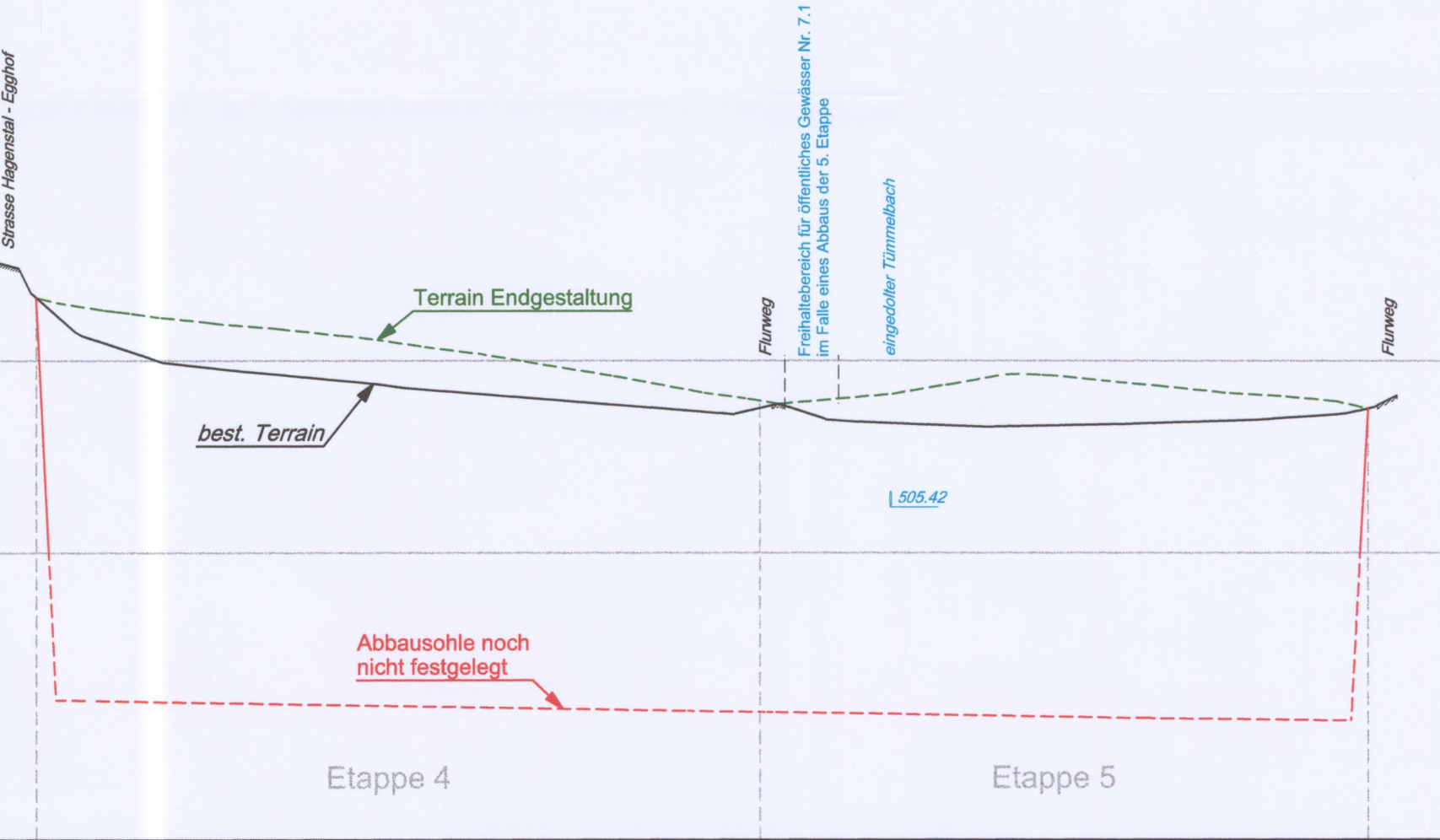
Schnitt 3 - 3
