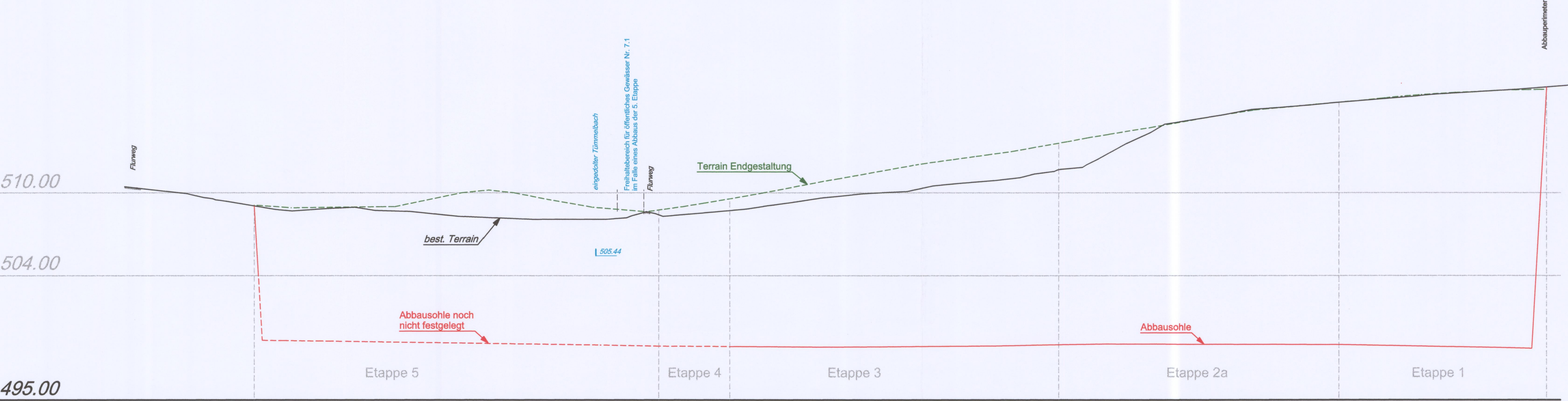
Schnitt 1 - 1
