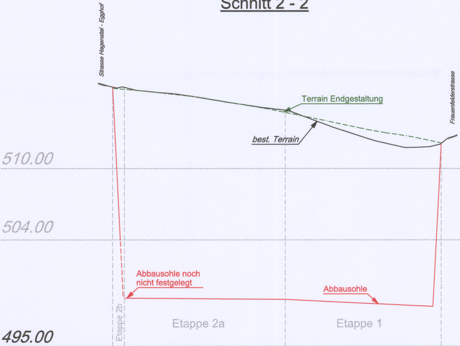
Schnitt 2 - 2
