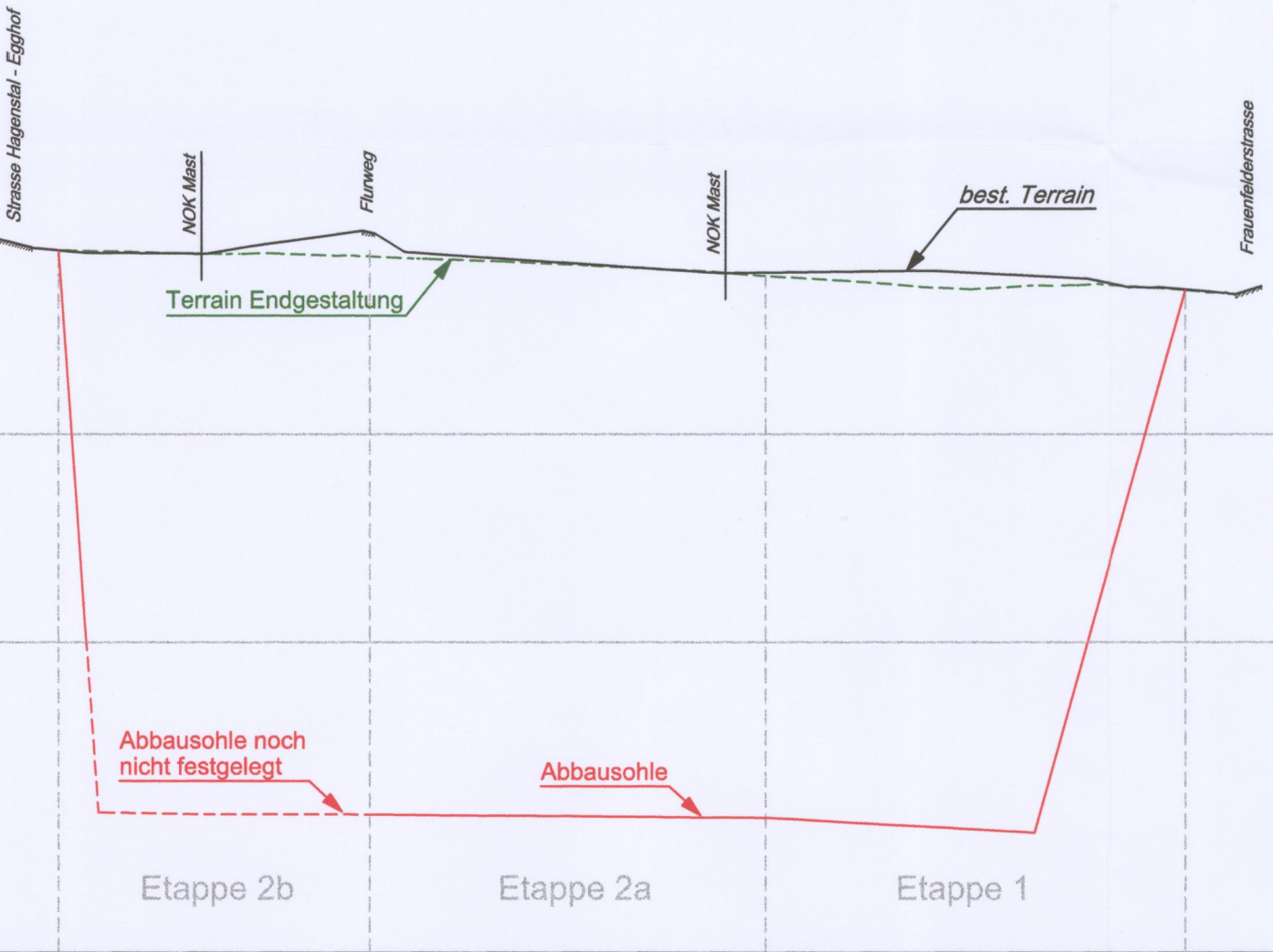
Schnitt 2a - 2a
