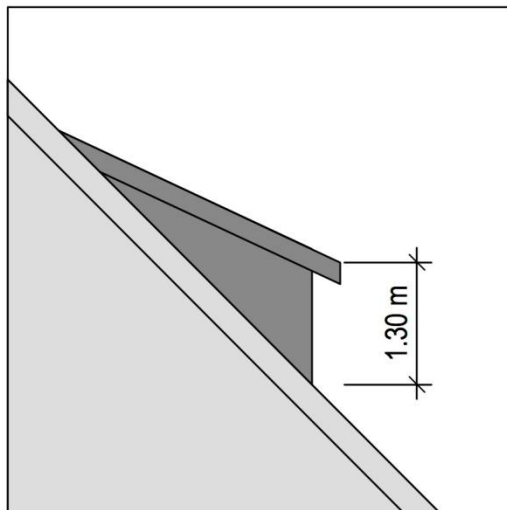
Seitenansicht, max. Fronthöhe
